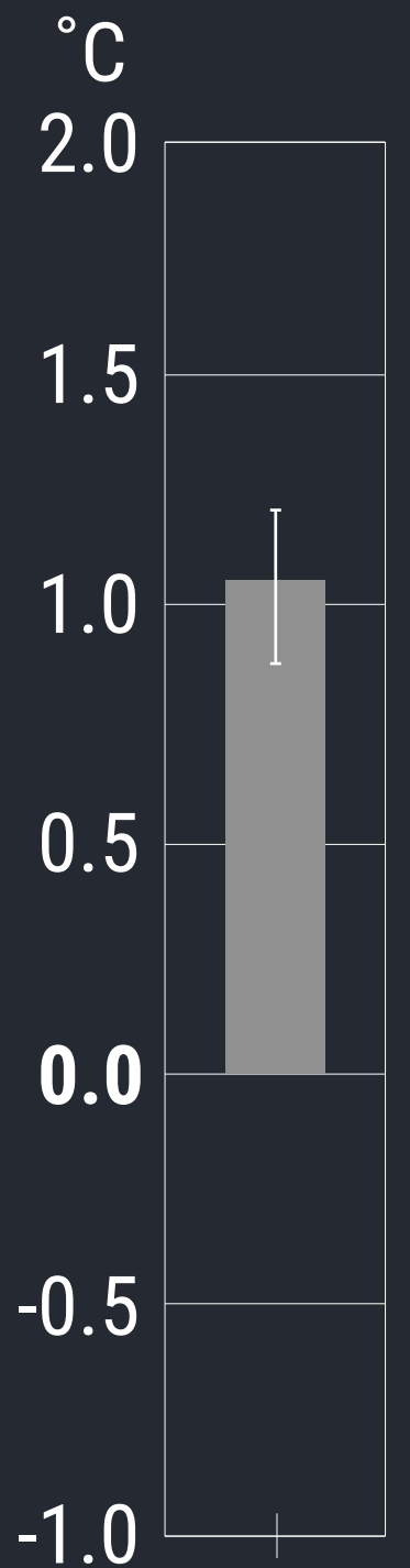
Încălzirea observată 2010–2019 față de 1850–1900
