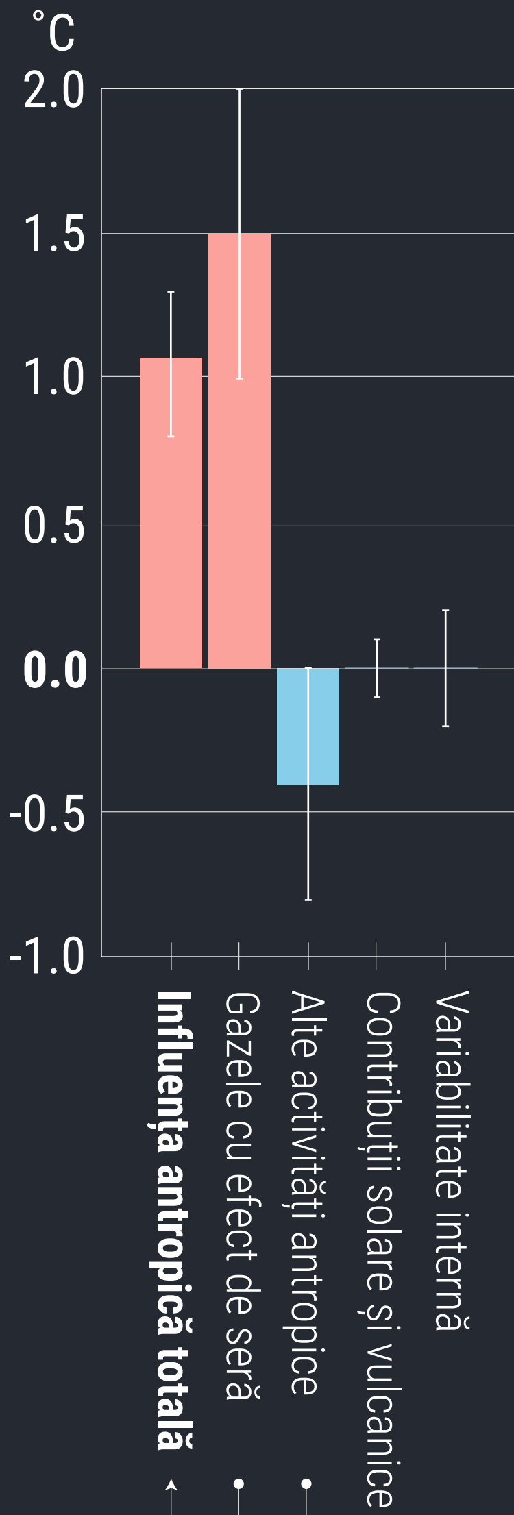
Contribuții la încălzirea 2010–2019 față de 1850–1900 din studii de atribuire
