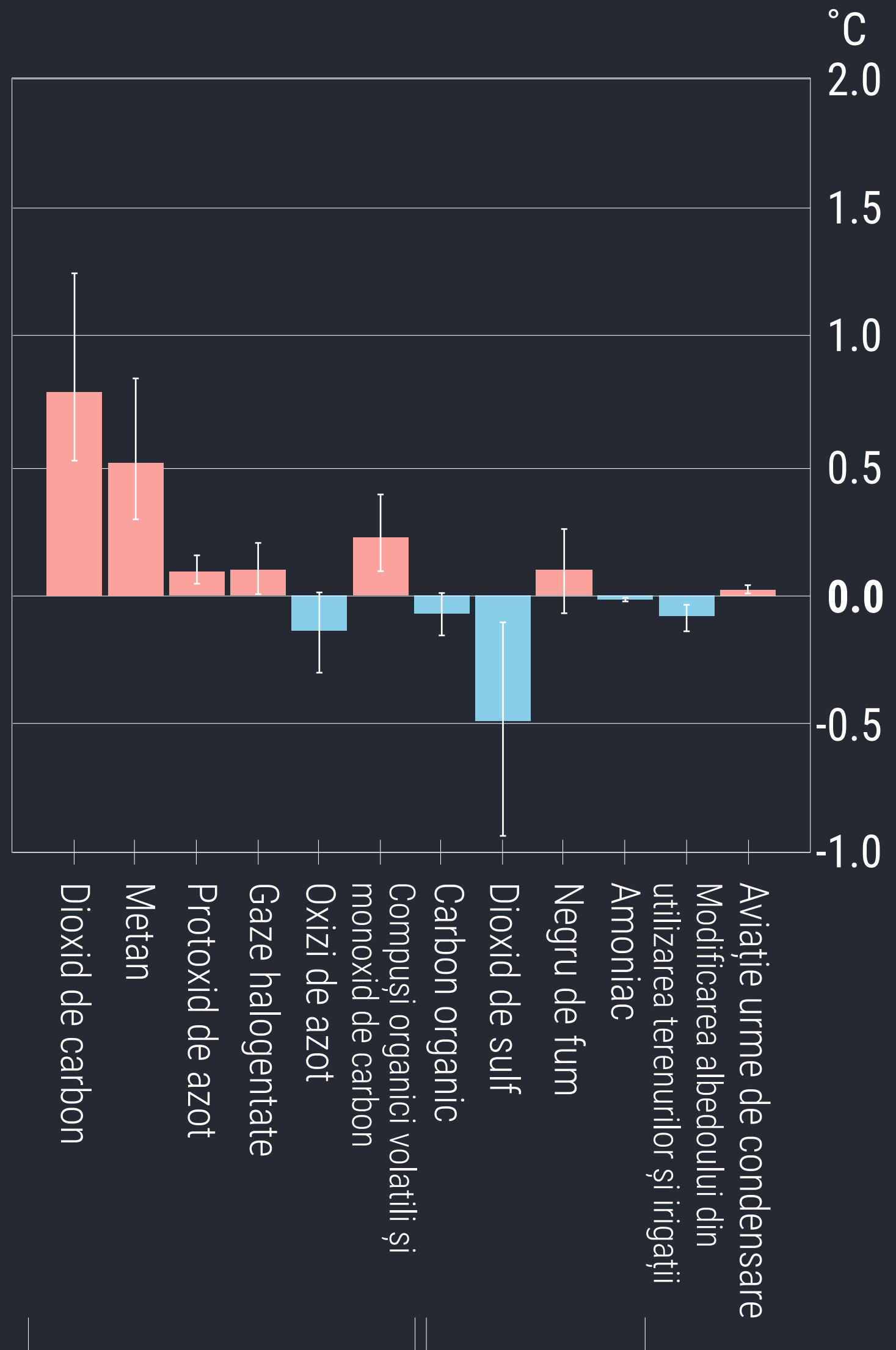
Contribuții la încălzirea 2010–2019 față de 1850–1900 din studii de forcing radiativ
